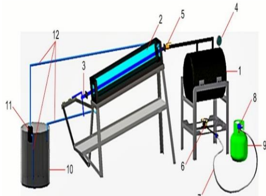
Gambar 4. Instalasi Peralatan Pengujian Keterangan gambar :
