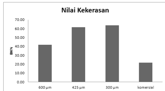
Gambar 3. Nilai kekerasan kampas rem komposit epoxy aluminium-serbuk tempurung kelapa
