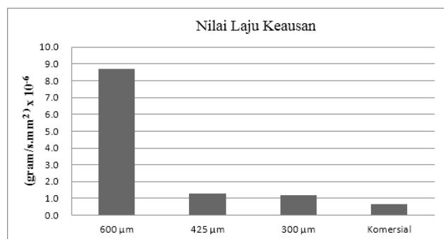
Gambar 4. Nilai laju keausan kanvas rem komposit epoxy aluminium-serbuk tempurung kelapa
