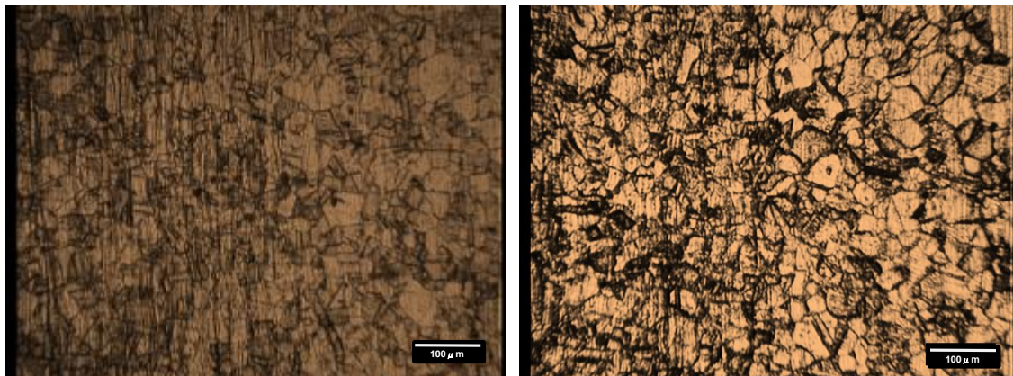
Gambar 4 Struktur mikro AISI 316L Setelah mengalami proses ball peening dengan tekanan (a) 6 bar (b) 8 bar
