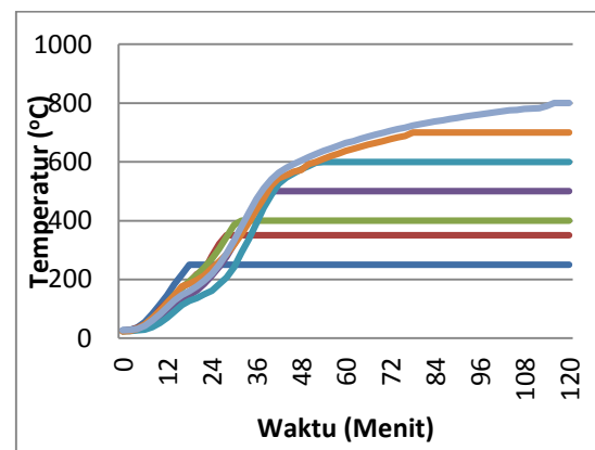
Gambar 3 Grafik Hubungan antara Waktu terhadap Temperatur Pirolisis
