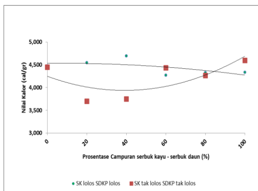
Gambar 2. Grafik hubungan antara nilai kalor dan prosentase campuran serbuk briket.
