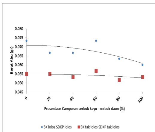
Gambar 3. Grafik hubungan antara berat abu dan prosentase campuran serbuk briket.
