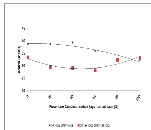
Gambar 4. Grafik hubungan antara waktu pembakaran dan prosentase campuran serbuk briket.
