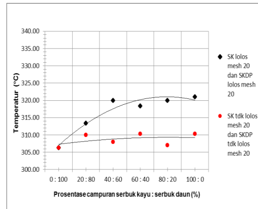
Gambar 6. Grafik hubungan prosentase campuran serbuk dan temperature briket
