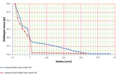
Gambar 5. Grafik hubungan prosentase campuran serbuk dan kecepatan penurunan massa briket
