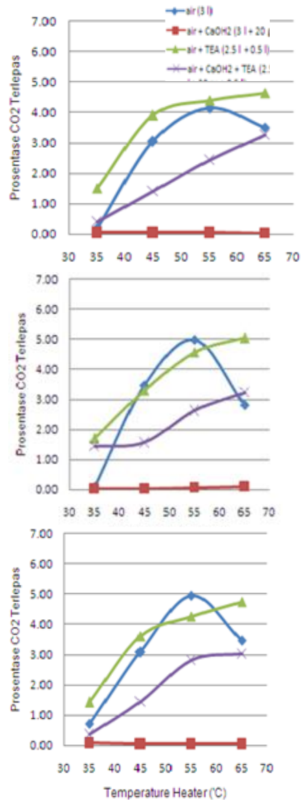
Gambar 3. Hubungan Temperatur terhadap Persentase CO 2 Terlepas diheater pada konsentrasi CO 2
