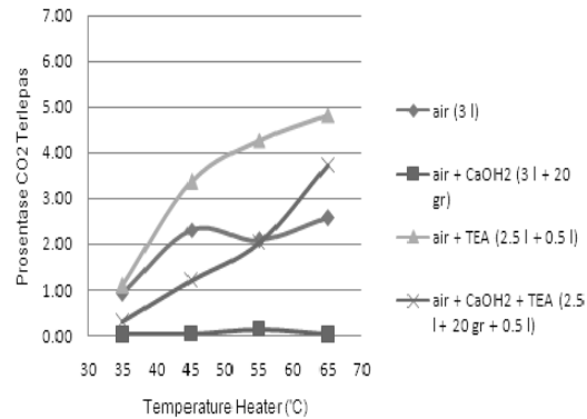
Gambar 2. Hubungan Temperatur terhadap persentase CO 2 Terlepas diheater pada konsentrasi CO 2 yang masuk 5%.
