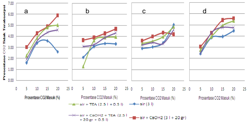
Gambar 4. Hubungan Persentase CO 2 tidak terabsorpsi dipacked collum terhadap Persentase CO 2 masuk pada Temperatur (a)35°C, (b)45°C, (c) 55°C dan (d) 65°C
