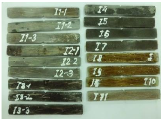
Gambar 9. Spesimen Uji Impak
